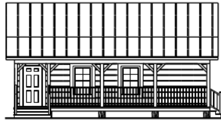
FRONT ELEVATION SCALE: 1/8" = 1'-0"
