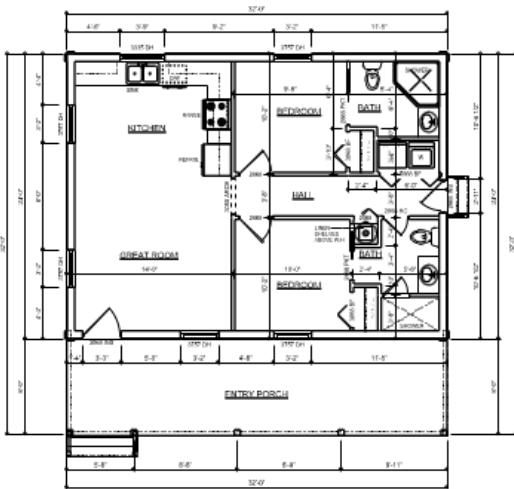
FLOOR PLAN SCALE: 1/8" = 1'-0"
